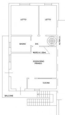
PIANO PRIMO H. 2.80
